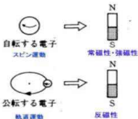
図1 磁性の起源
