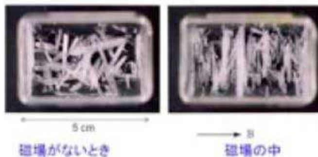
図3 ベンゾフェノン結晶の磁気配向
