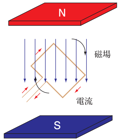
発電機の原理
