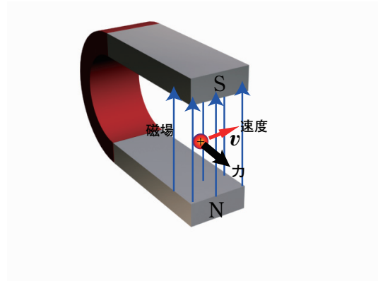
移動する電荷は磁場により力を受ける
