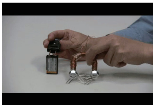
電磁石の実験
