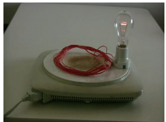
電磁誘導の実験
