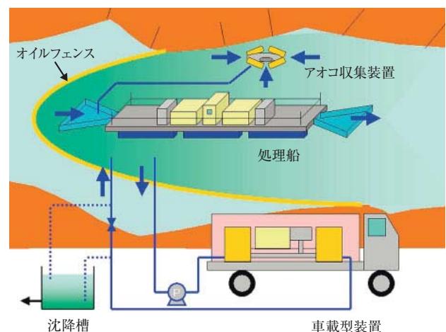
図1 装置設置例
