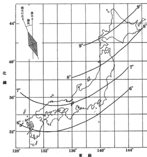
日本の偏角分布
