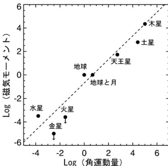
磁気ボーデの法則
