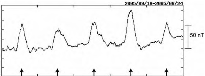
地磁気水平成分の日変化( グアム島 )。2005 年 9 月 19 日 - 23 日の 5 日間について示す ( 矢印は正午 )。
