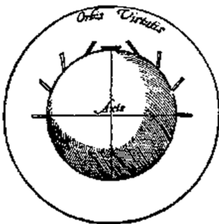
ギルバートの地磁気模型
