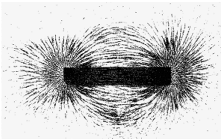
砂鉄の実験によって見える磁力線の形
